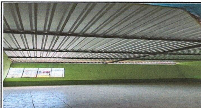
Foto 4: Cambio de lámina troquelada e instalación eléctrica en aulas
